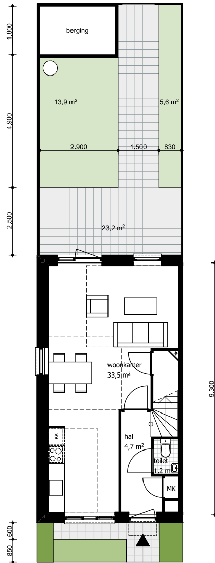
GO begane grond 43,7 m 2
