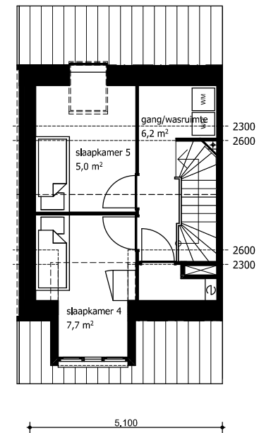
GO 2e verdieping 30,6 m 2
