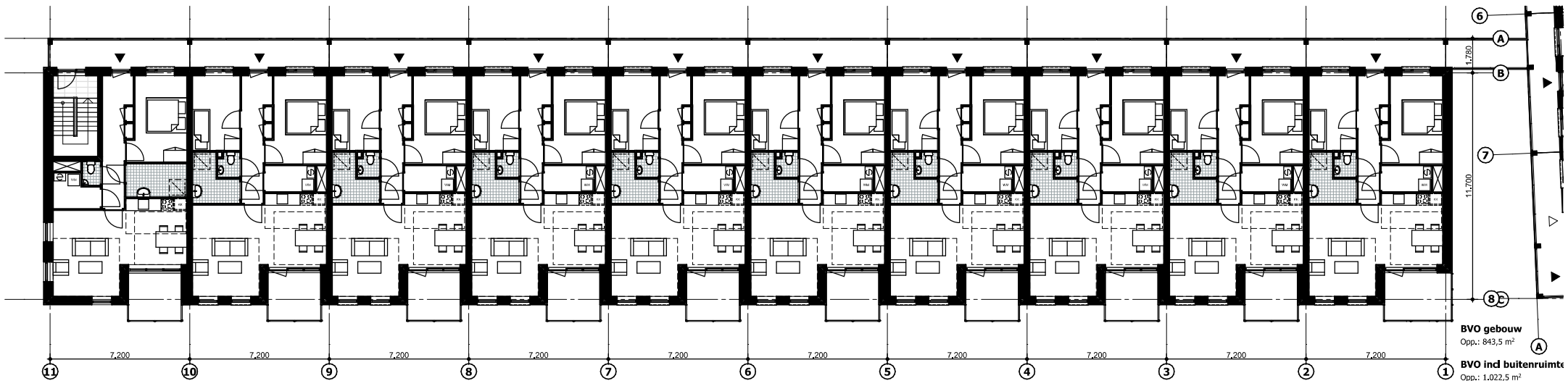
2e verdieping
